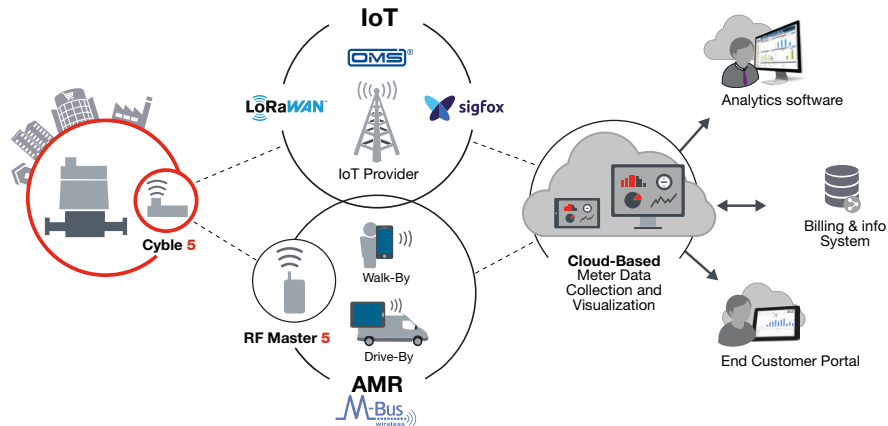
Sistem Internet of Things (IoT) dan AMR menggunakan modul Cyble
