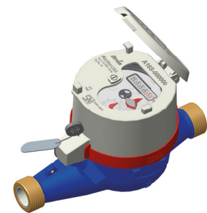
Multimag TMII Cyble R50
